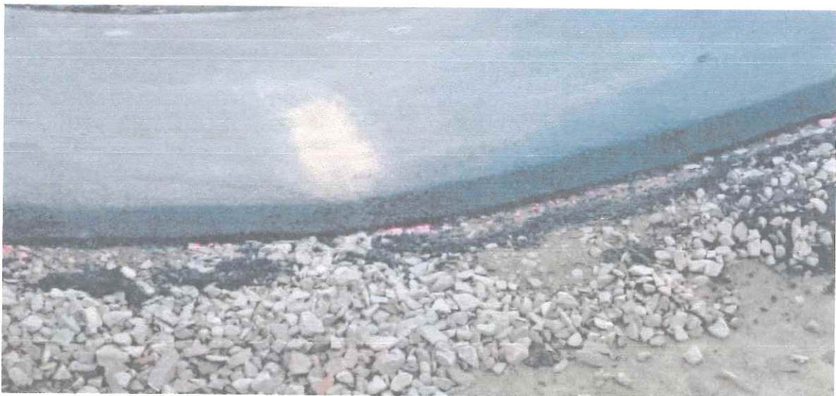
Prawidłowo zagęszczona i wyprofilowana nawierzchnia asfaltowa
